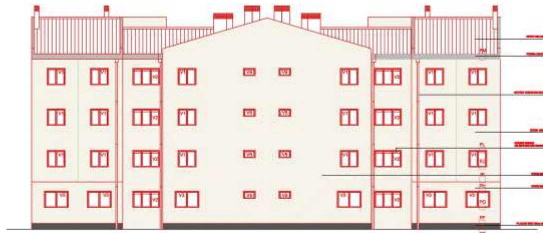
ALÇADO POSTERIOR BLOCOS 6/9/30
