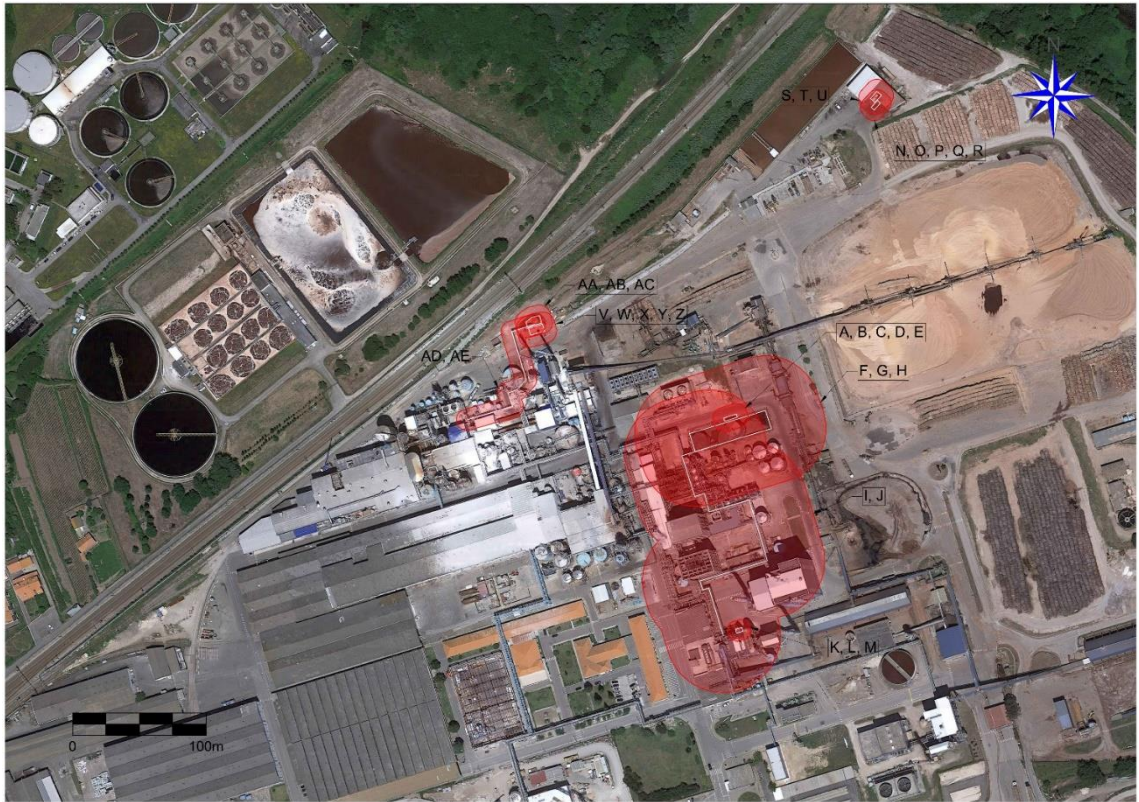
Figura 3: Alcances dos cenários mais gravosos para a radiação de 12,5 kw/m²
