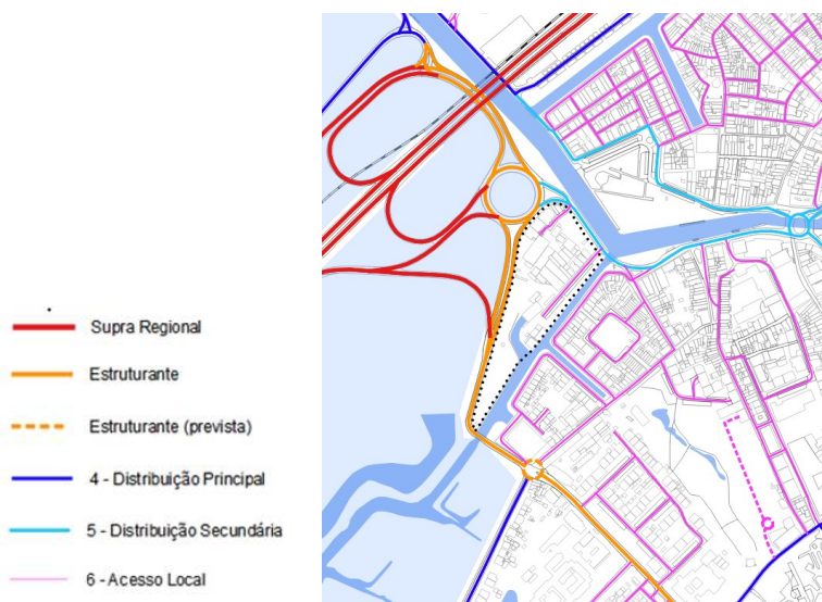
Figura 6 Extrato da carta de hierarquia viária – PDM- 1ª revisão
