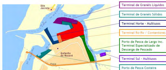
Figura 83 – Planta Geral do Porto de Aveiro
